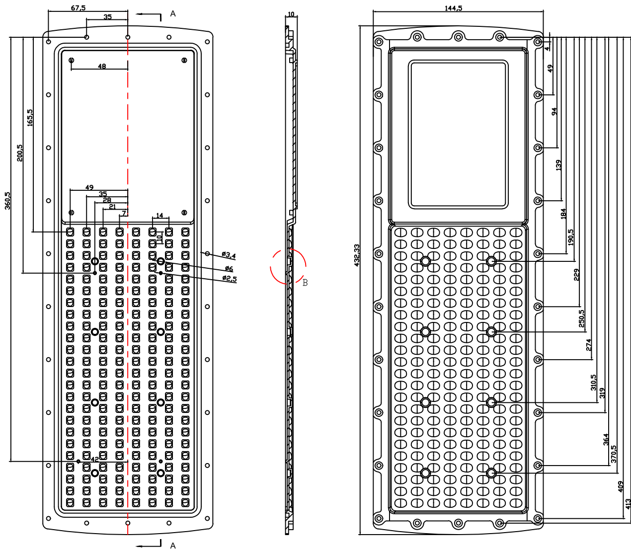
SECTION A-A
