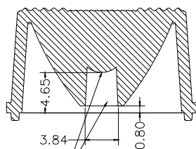
发光孔侧面一截及球面晒雾纹
