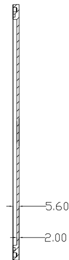
SECTION A-A
