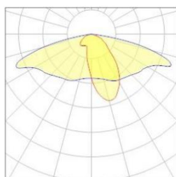
S01.01.02.423 MAXWELL-8-LN_3535
