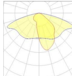
S01.01.02.444 MAXWELL-8-SCL_3535
