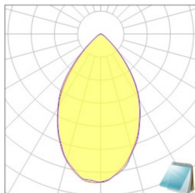
S01.01.01.337 MAXWELL-8-60_3535
