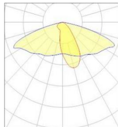
S01.01.02.458 MAXWELL-8-LN2_3535
