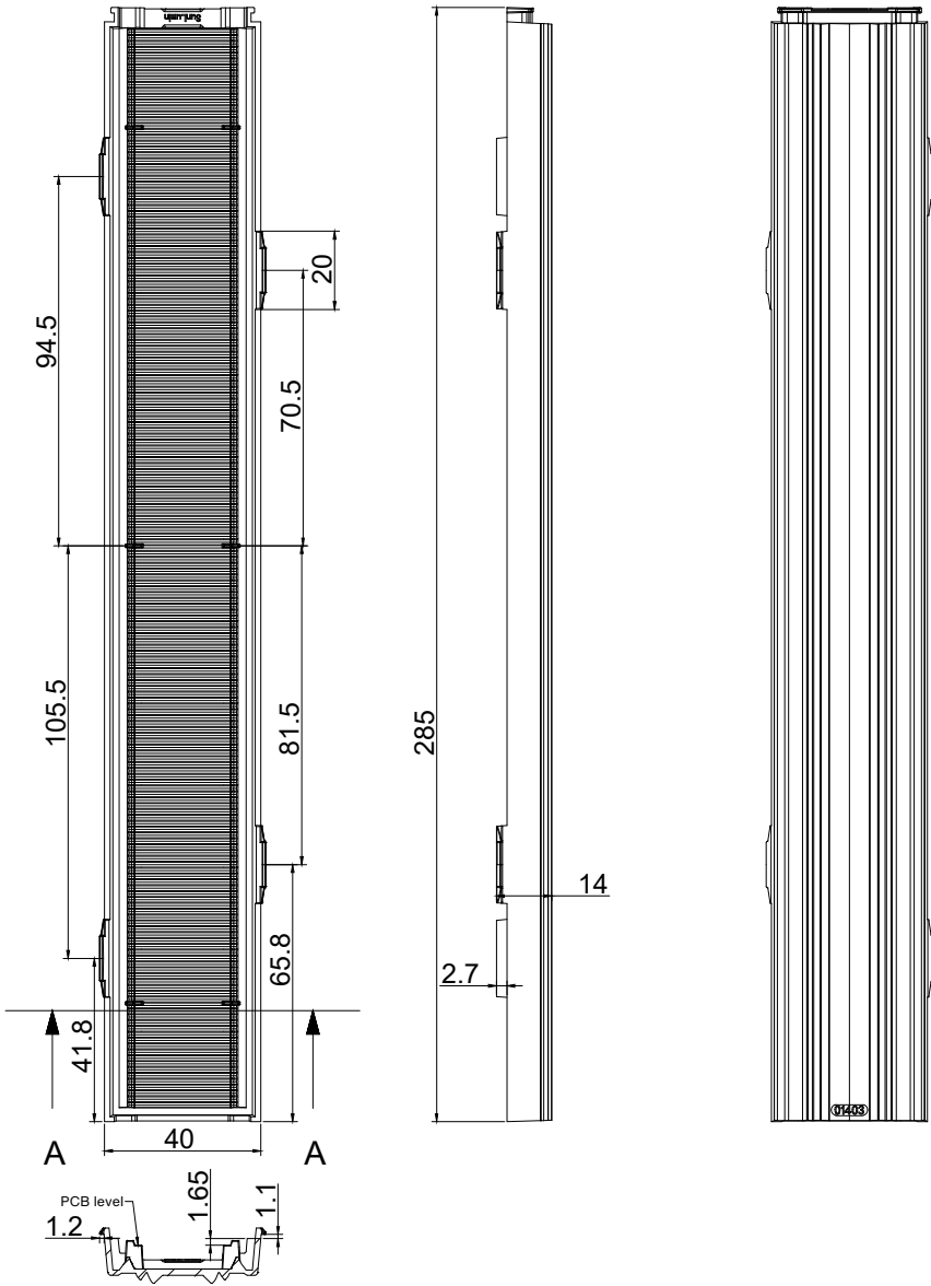
SECTION A-A
