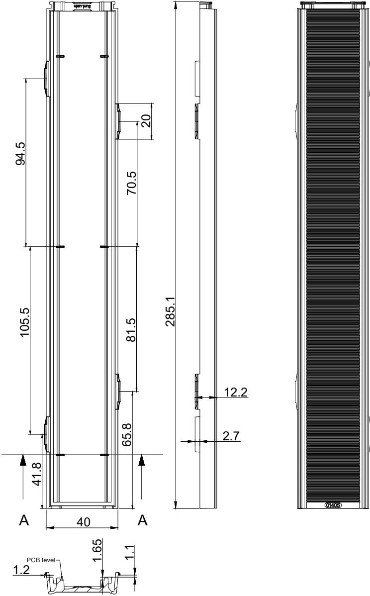
SECTION A-A
