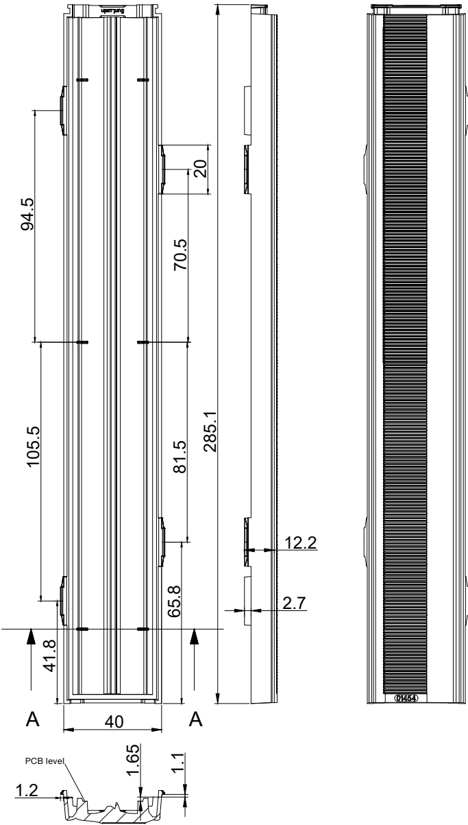
SECTION A-A
