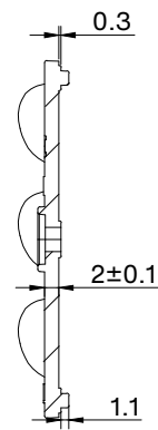
SECTION A-A
