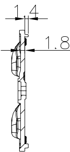
SECTION A-A
